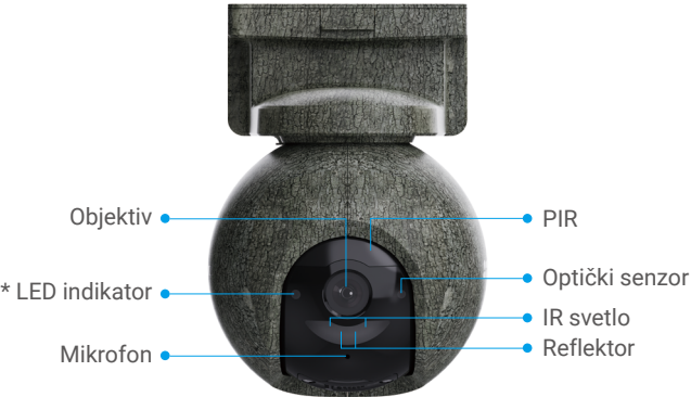
Prednji prikaz
